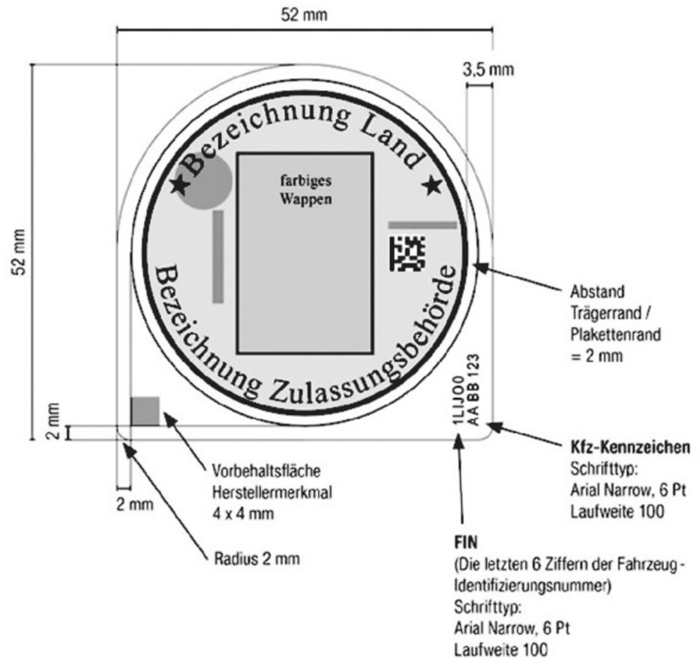
Abbildung 3: Bemaßung des Plakettenträgers
